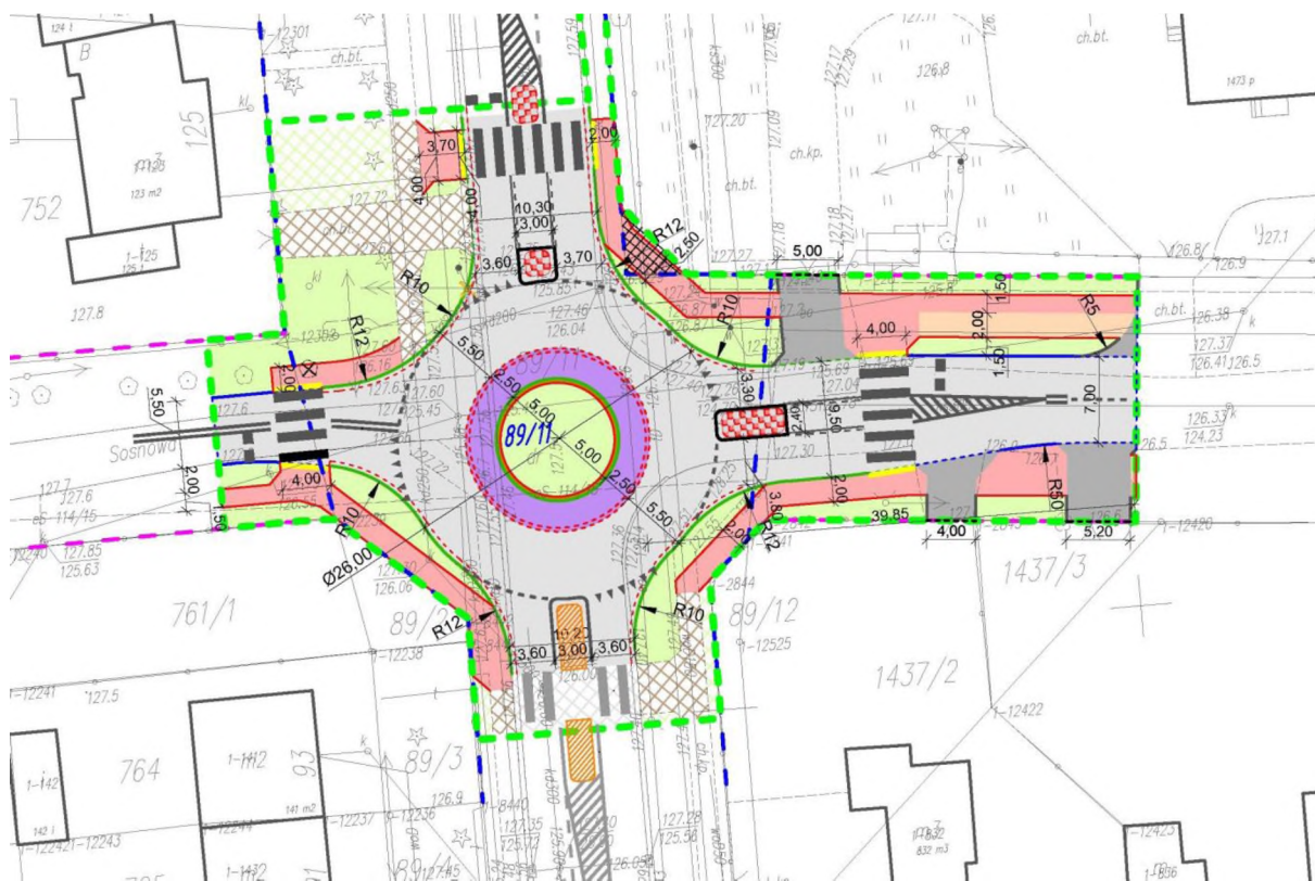
Ryc. Plan ronda mającego być zrealizowanym w ramach zadania „Rozbudowa istniejącego skrzyżowaniu w ciągu drogi krajowej nr 57- na skrzyżowaniu ul. Grunwaldzkiej z ul. Brzozową, na skrzyżowanie o ruchu okrężnym oraz włączenie do niego ul. Sosnowej w miejscowości Chorzele, źródło Urząd Miasta i Gminy w Chorzelach
