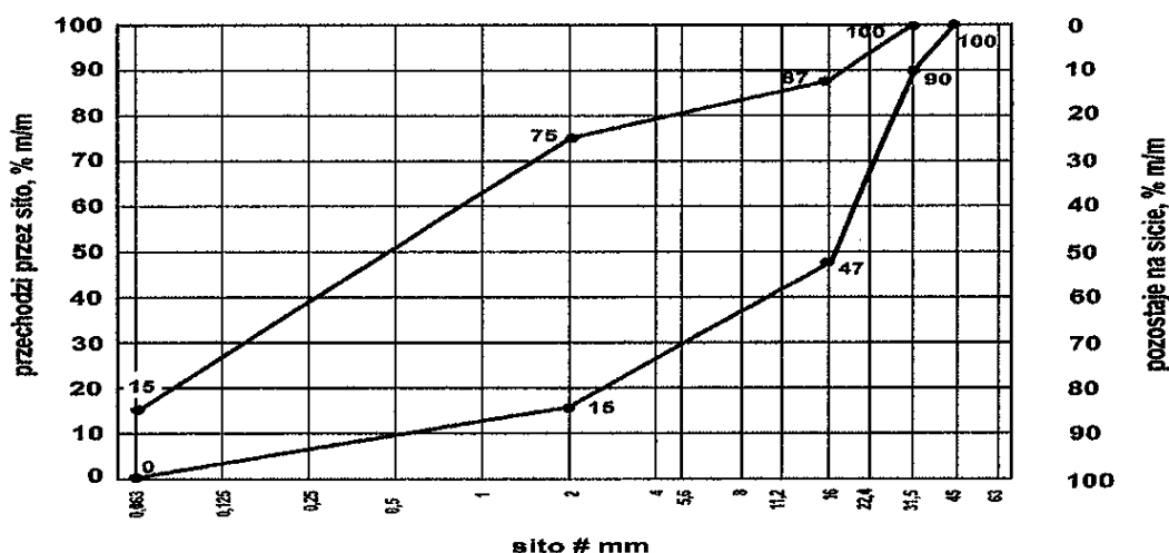
Rys. 1. Krzywe graniczne uziarnienia mieszanki kruszywo niezwiązanej 0/31,5 mm do nawierzchni
